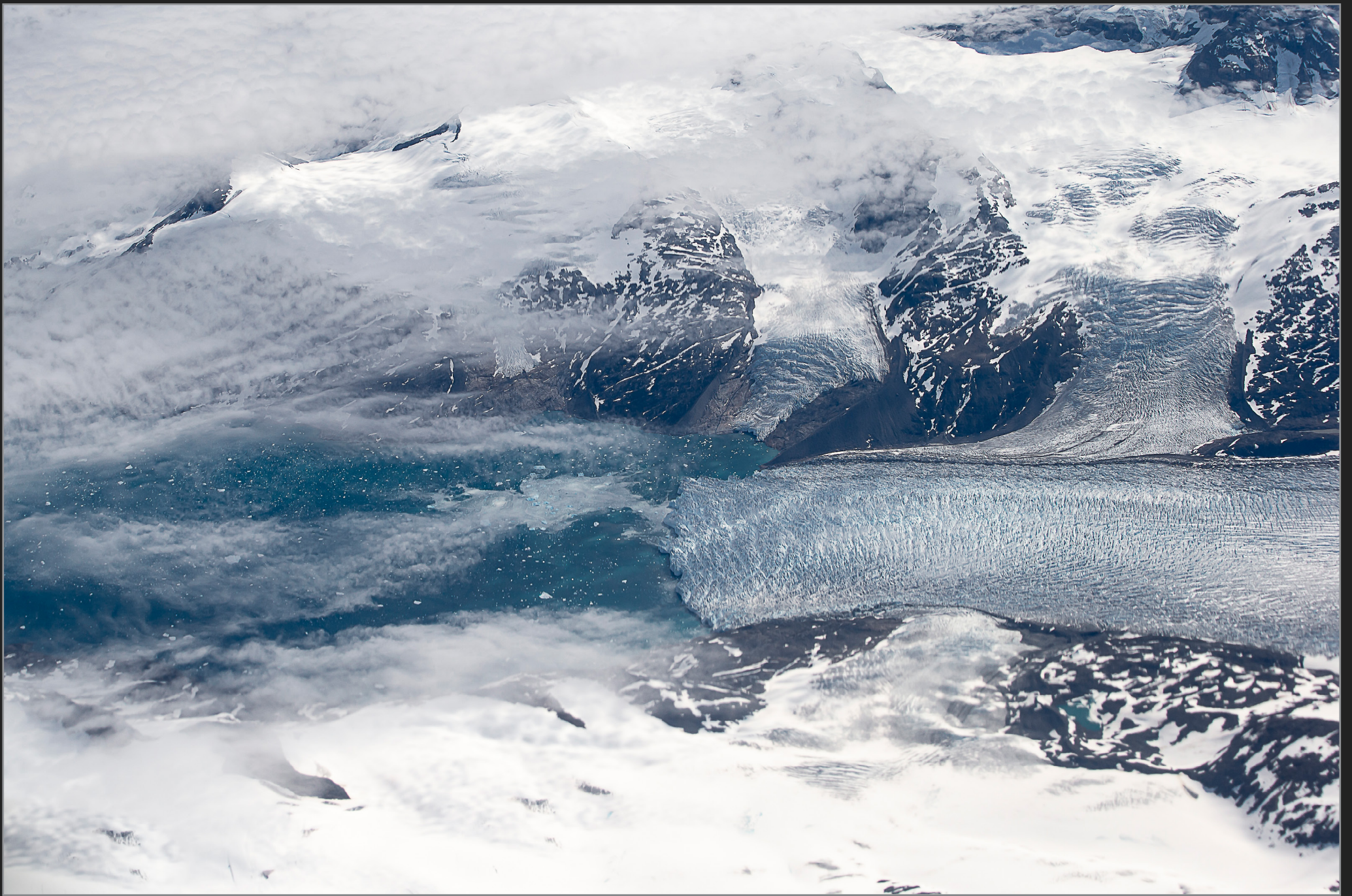
Sydgrønland, juli 2016
